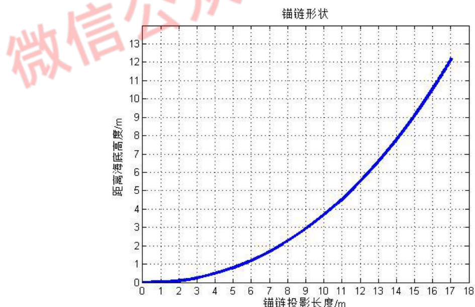
图 7 海面风速为 24m/s 时锚链形状图形
